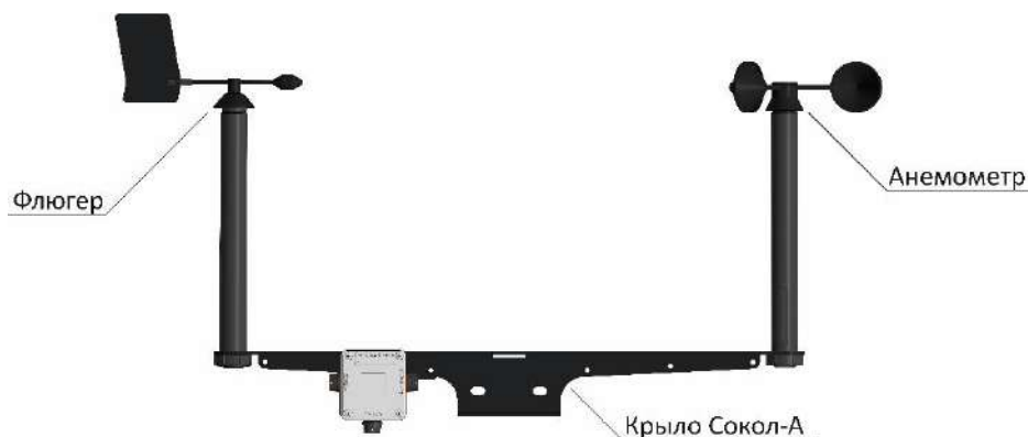
Рисунок 1–Внешний вид анеморумбометра СОКОЛ–А
